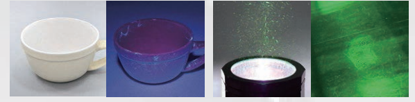
365紫外線レンズカバー 型式:3050BL365S-LC 530粉塵調査レンズカバー 型式:3050GD530-LC 拡散365紫外線レンズカバー 型式:3050BL365W-LC
